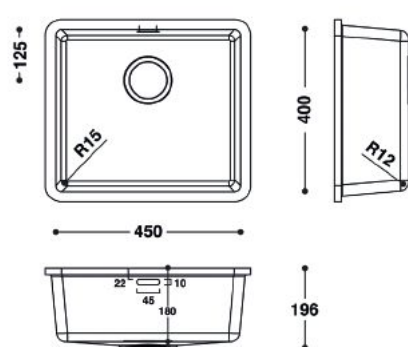
CS454 450 X 400 X 180 mm
