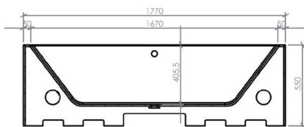
COUPE A-A
