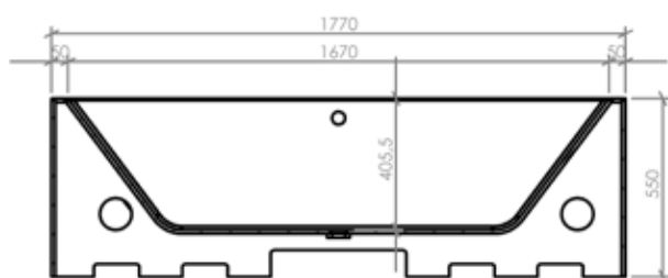
COUPE A-A
